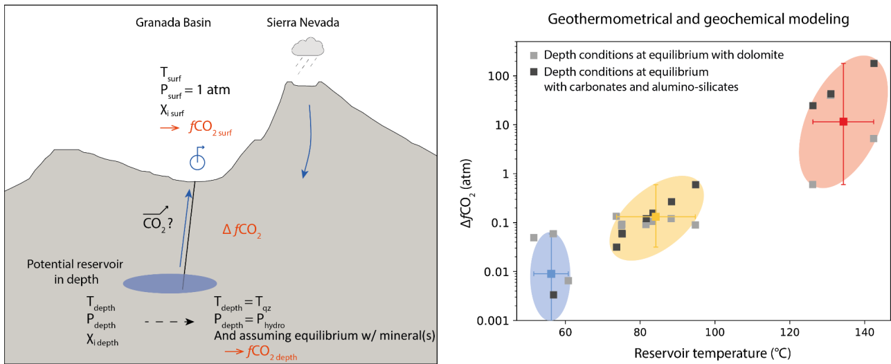
Figure 1 - Représentation schématique et graphique des modélisations géothermiques et géochimiques réalisées sur les sources thermales de la Cordillère Bétique.
