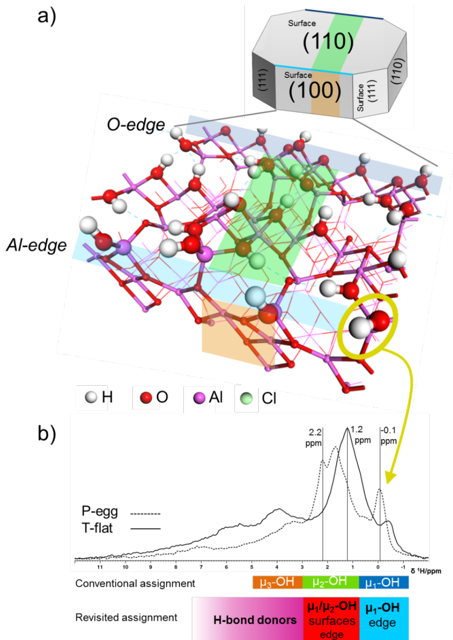
Figure : a) Cristallite d'alumine gamma et détail du modèle d'arête ; b) Spectre RMN du proton des deux aluminas étudiées (P-egg, morphologie avec beaucoup d'arêtes et T-flat avec peu d'arêtes), l'attribution de ces signaux dans la littérature jusqu'à présent et l'attribution révisée proposée dans [1].
