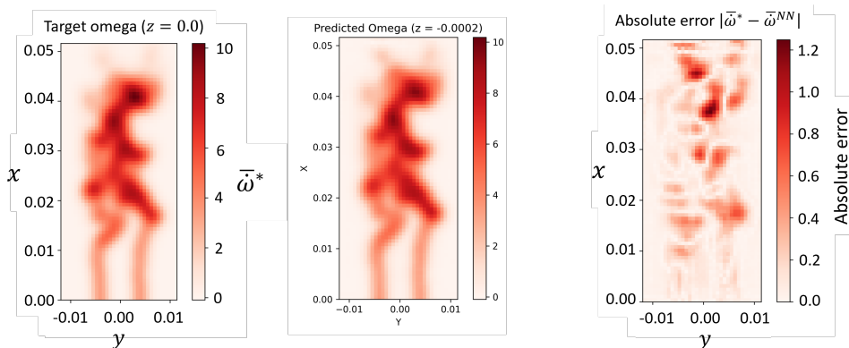
Figure 1: comparaison du taux de réaction d'hydrogène \omega (mol/s) entre une solution de référence (gauche) et un champ prédit par CNN (centre). L'erreur absolue entre les deux champs est représentée à droite
