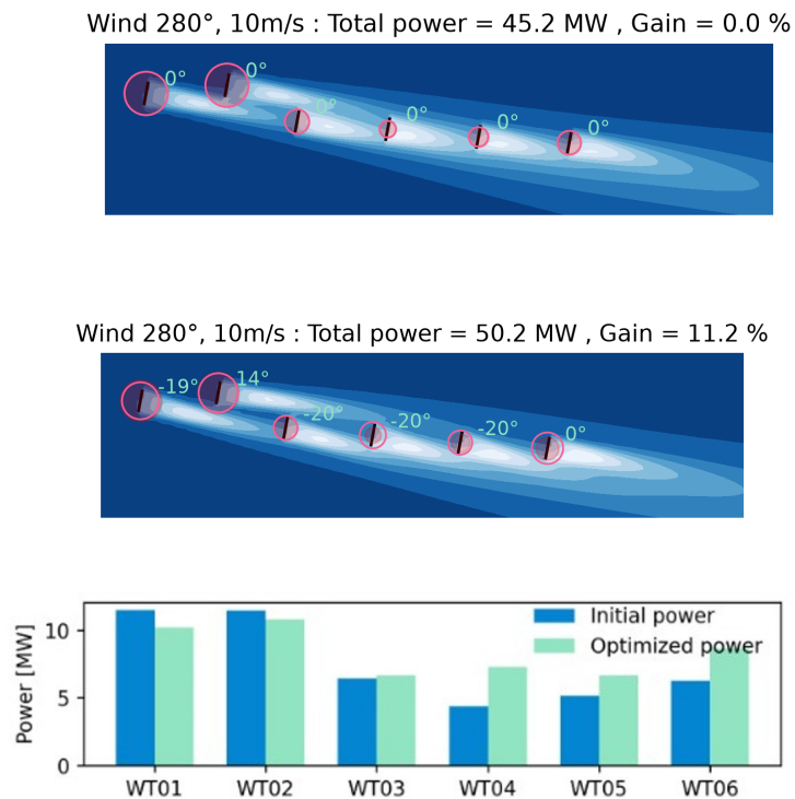
Figure 3. Le contrôle par redirection de sillage permet d'augmenter la production totale d'un parc éolien (la taille du cercle rouge est proportionnelle à la production de l'éolienne).
