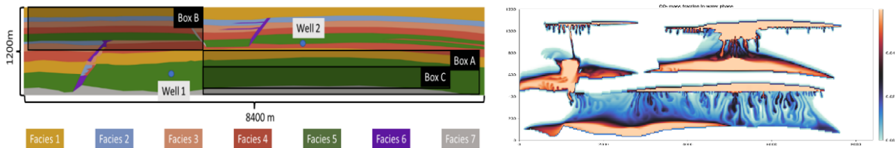
Figure 1 : Distribution des facies lithologiques dans le réservoir et emplacement des puits injecteurs Well1 et Well2 (à gauche), distribution finale du CO 2 dissous dans l'eau obtenue avec le simulateur d'IFPEN : Geoxim (à droite)
