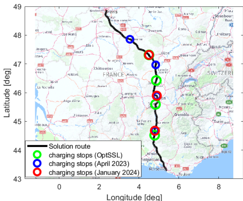
Figure 2 : Solutions optimales d'itinéraire pour un trajet de Paris à Marseille avec trois configurations d'IRVE : infrastructure existante en avril 2023, infrastructure existante en janvier 2024, infrastructure optimale calculée par notre méthode (OptSSL). Pour ce cas d'étude, notre solution optimale permet d'économiser jusqu'à 22 heures de temps de trajet par rapport à la configuration d'avril 2023 (contre seulement 6 heures économisées par la configuration de janvier 2024) pour un taux de véhicules électriques de 2% sur le flux véhiculaire total.
