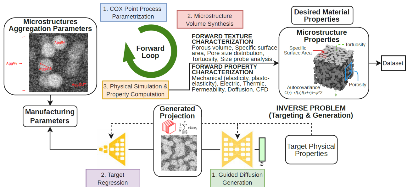
Figure 1 : boucle de co-conception des microstructures : en haut, boucle directe (forward loop) – synthèse des propriétés à partir des paramètres de fabrication ; en bas, boucle inverse – génération d'une microstructure à partir de propriétés cibles, puis retour aux paramètres de fabrication
