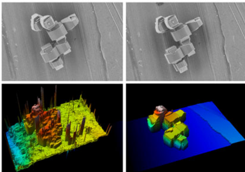
Reconstruction 3D d'une zéolithe.
