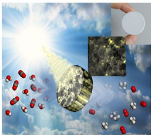
Photo-réduction en volume du \text{CO}_2 par des catalyseurs macrocellulaires monolithiques de type « \text{TiO}_2@\text{Si}(\text{HIPE}) ». Crédit : IFPEN
